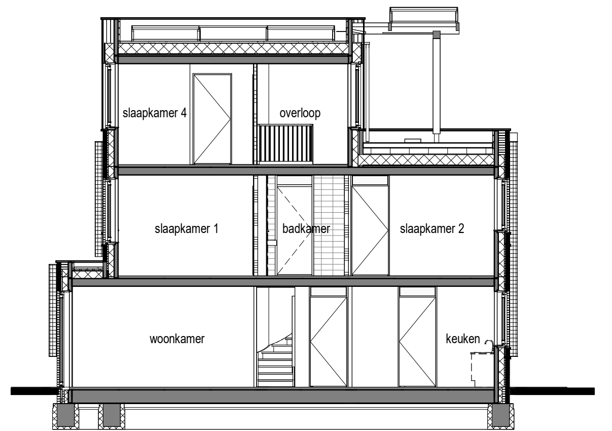
Doorsnede 1 : 100
