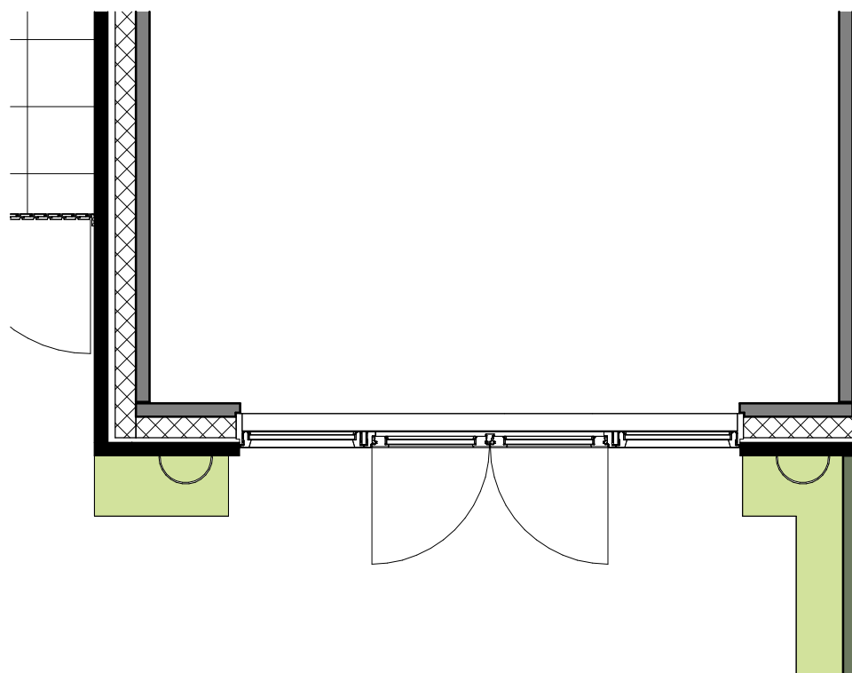
Begane grond 1 : 50
