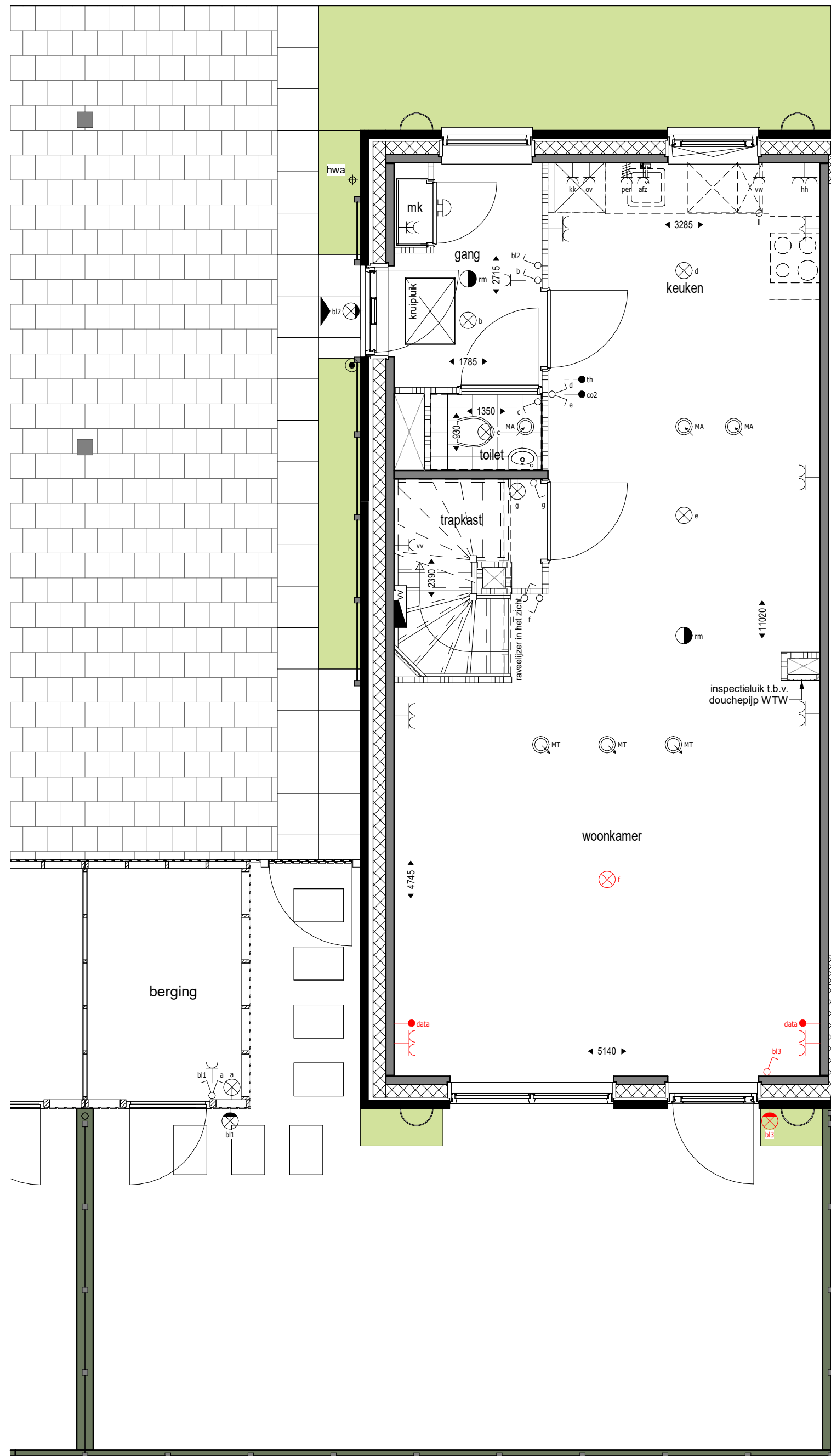
Begane grond 1 : 50
