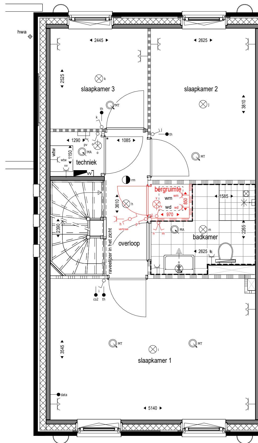
1 e verdieping 1 : 50
