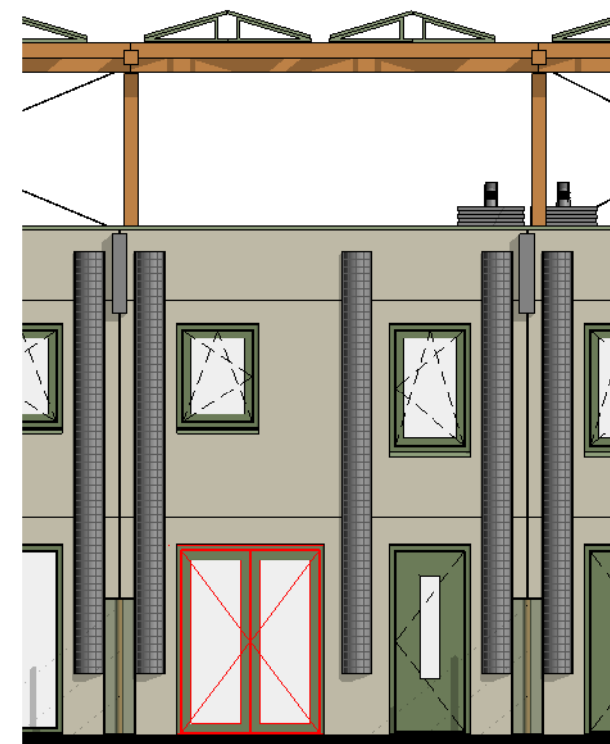
Voorgevel 1 : 100
