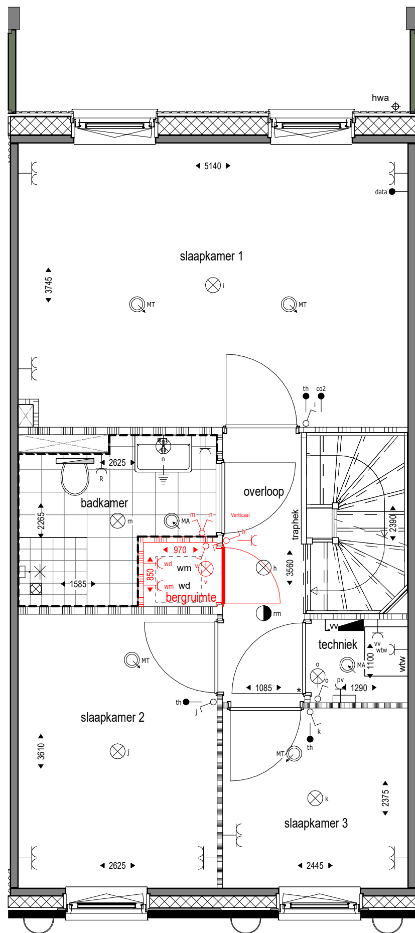
1 e verdieping 1 : 50
