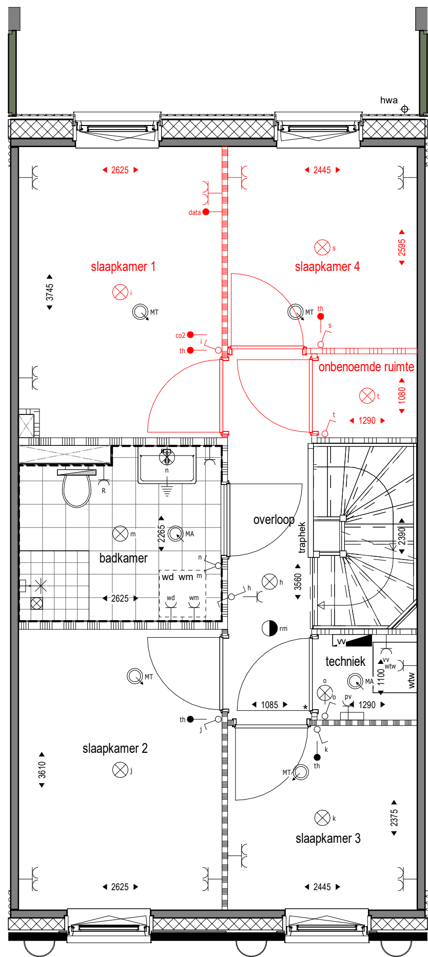
1 e verdieping 1 : 50
