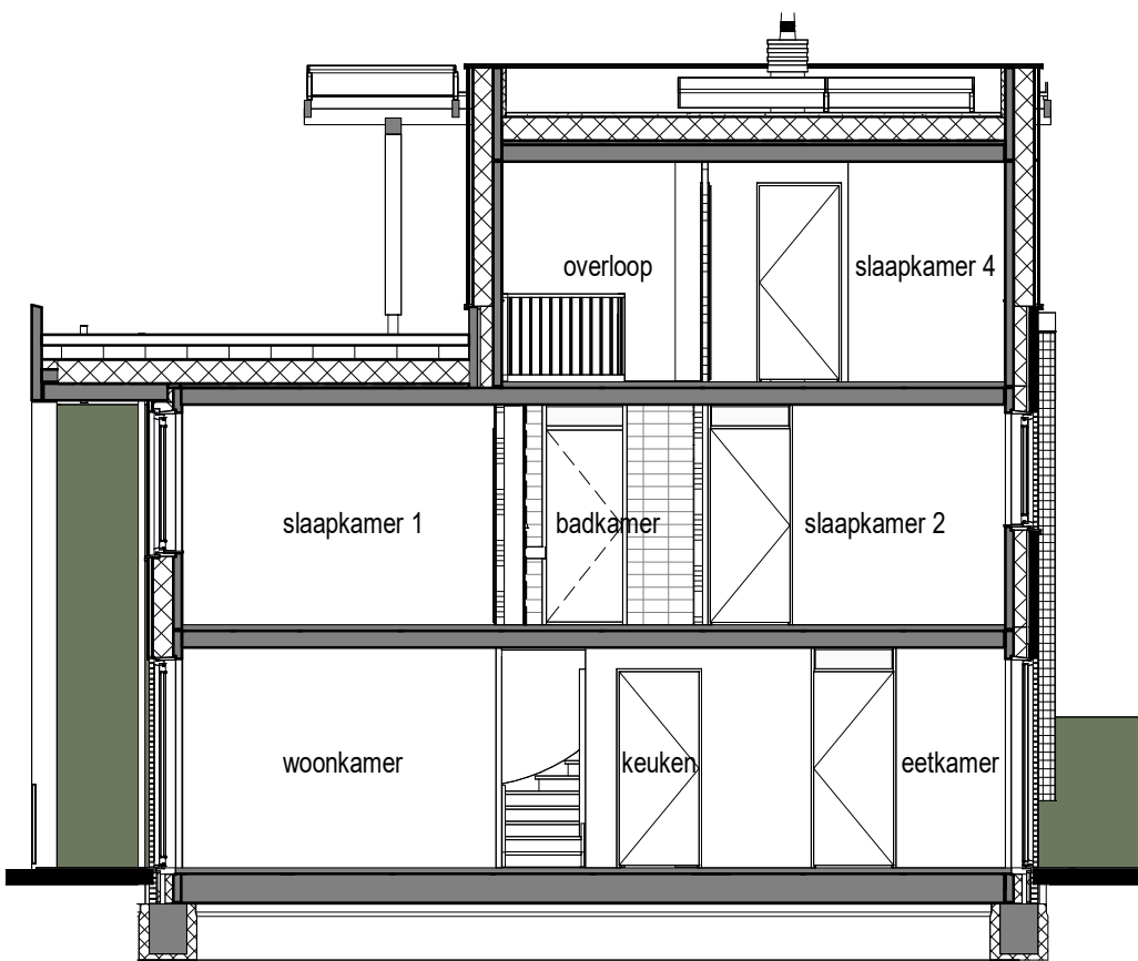
Doorsnede 1 : 100
