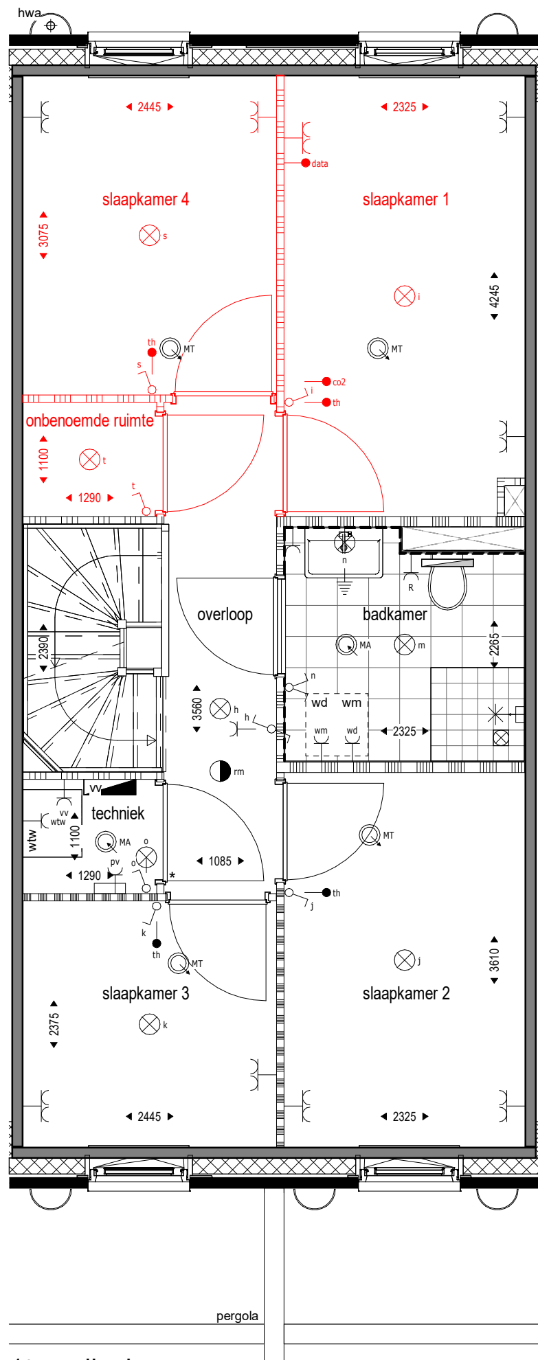
1e verdieping 1 : 50
