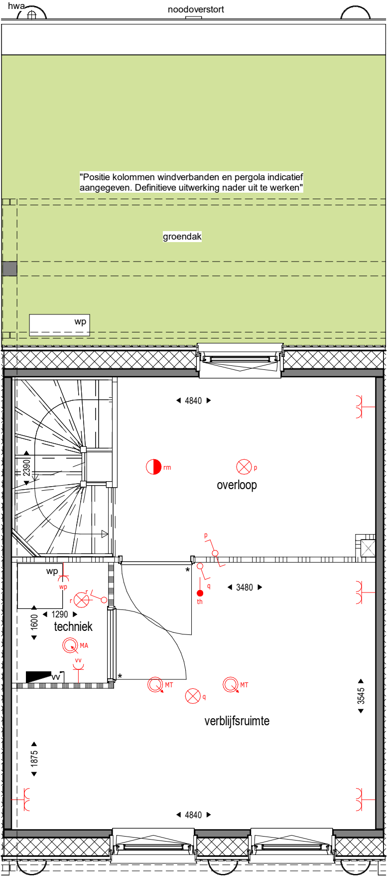
2e verdieping 1 : 50
