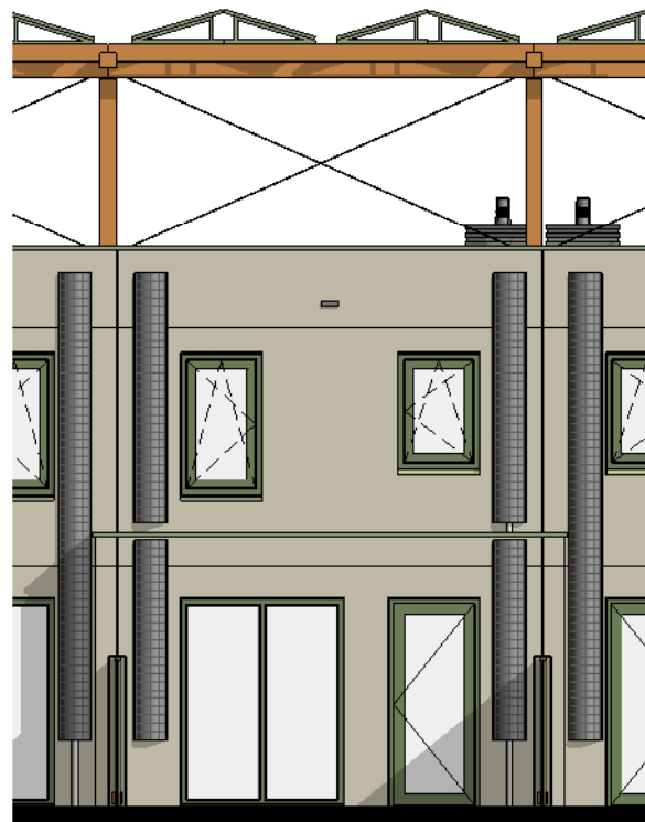
Achtergevel 1 : 10
