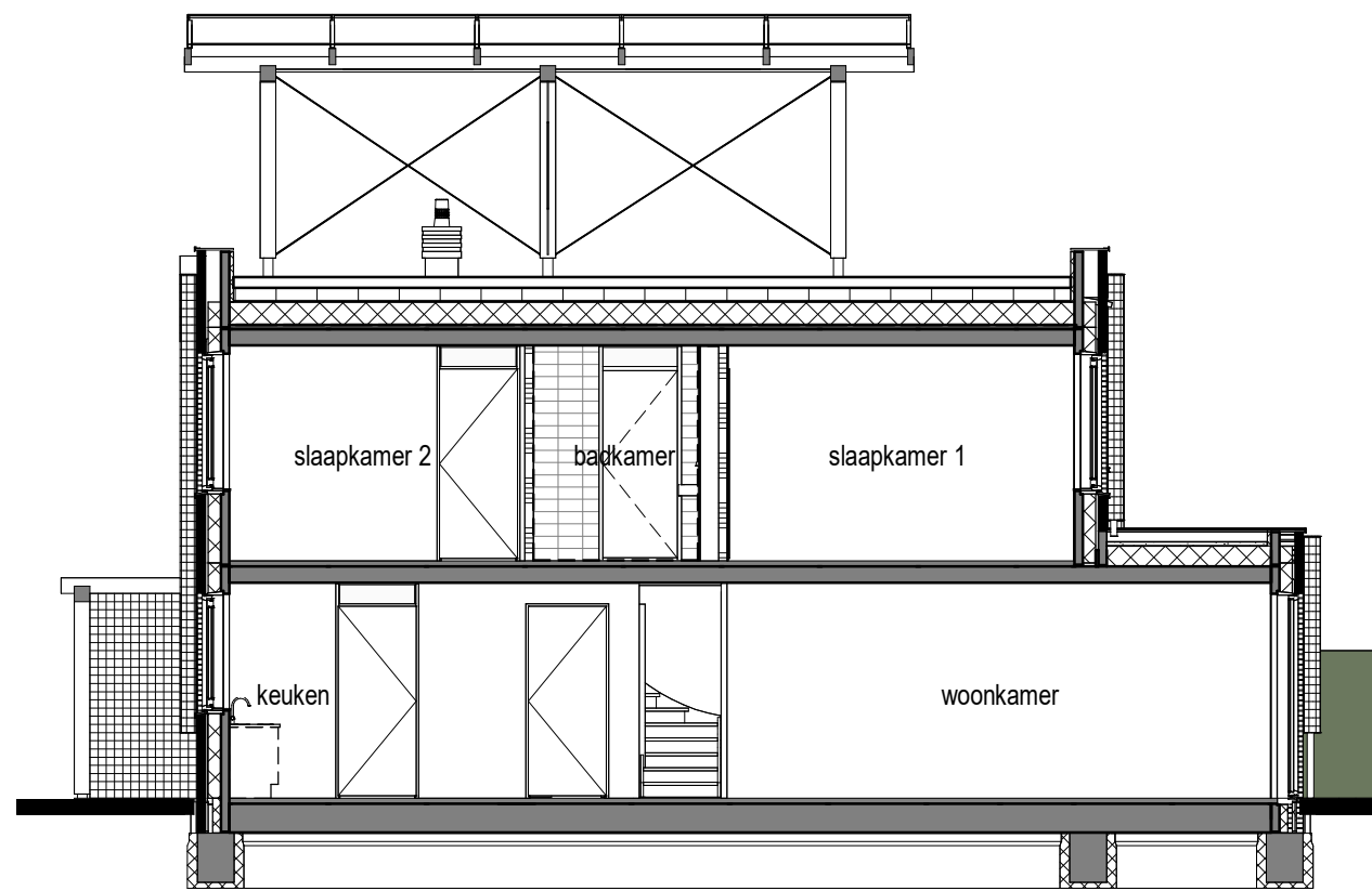
Doorsnede 1 : 100
