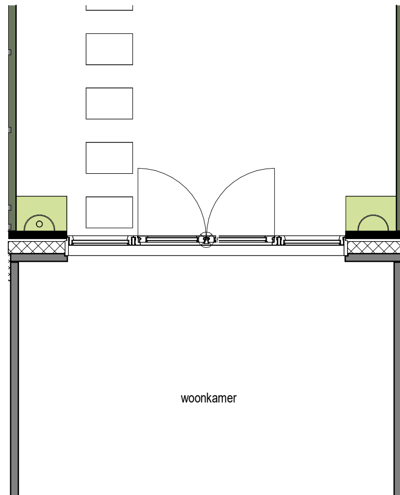
Begane grond 1 : 50
