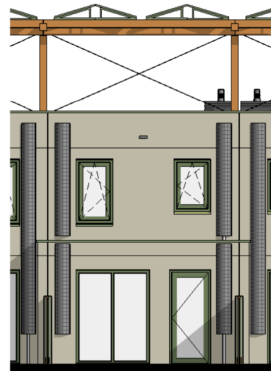
Achtergevel 1 : 10
