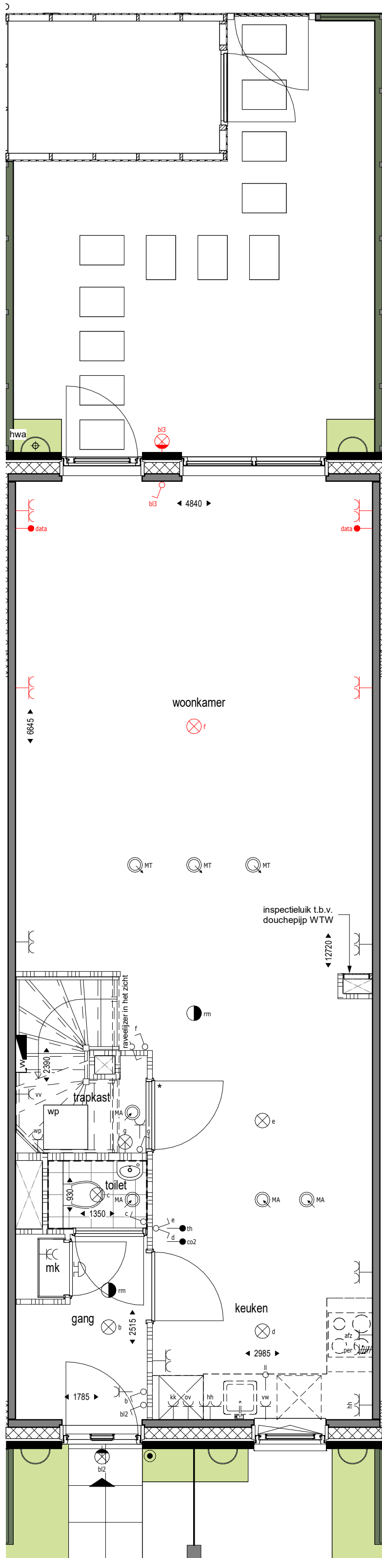
Begane grond 1 : 50
