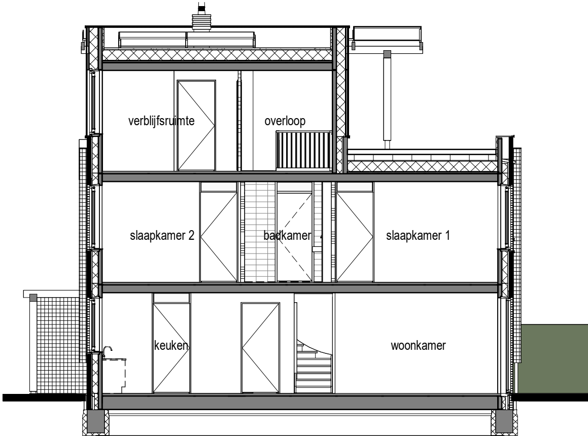
Doorsnede 1 : 100
