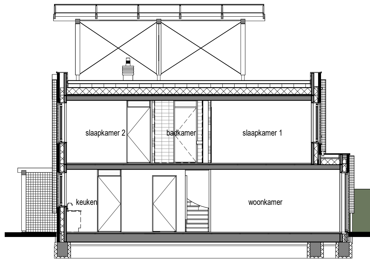
Doorsnede 1 : 100
