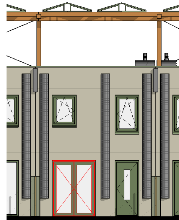
Voorgevel 1 : 100
