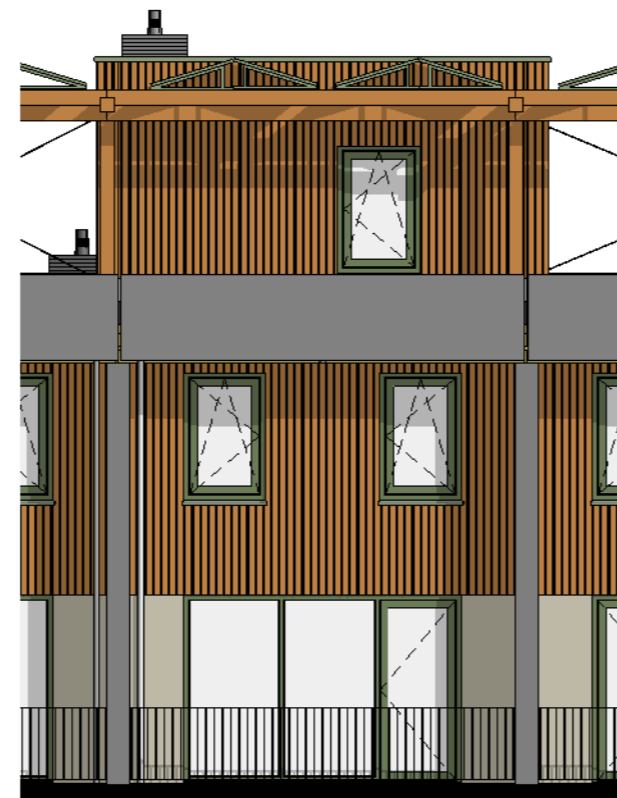
Achtergevel 1 : 100
