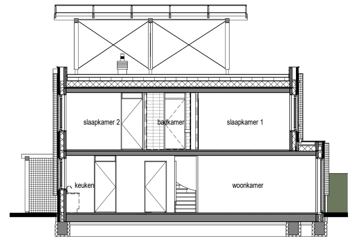
Doorsnede 1 : 100
