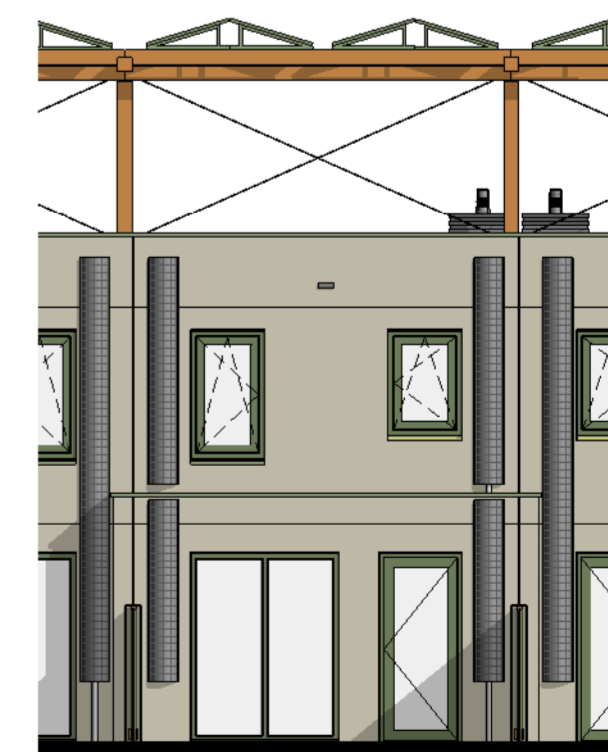
Achtergevel 1 : 10
