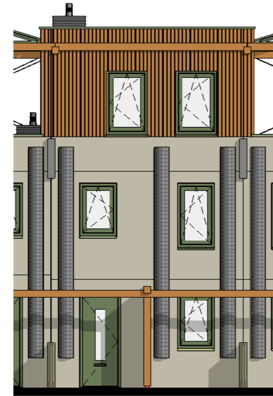
Voorgevel 1 : 100
