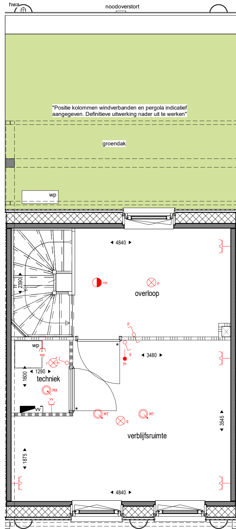
2 e verdieping 1 : 50
