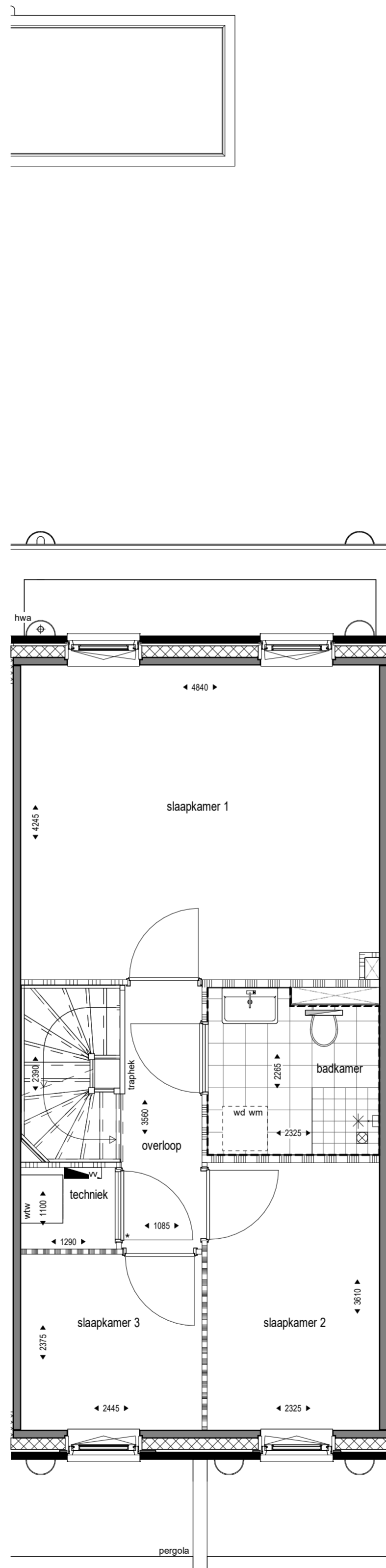
*Postie kolommen en pergola indicatief aangegeven. Definitieve uitwerking nader 1e verdieping 1 : 50
