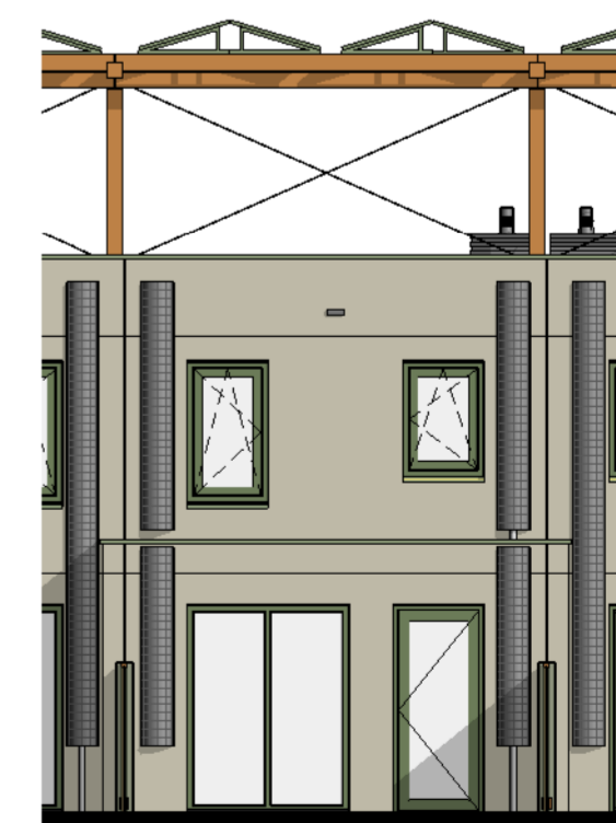
Achtergevel 1 : 10
