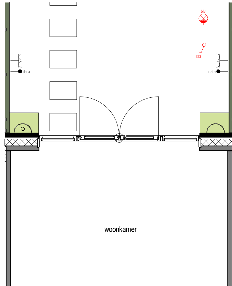
Begane grond 1 : 50
