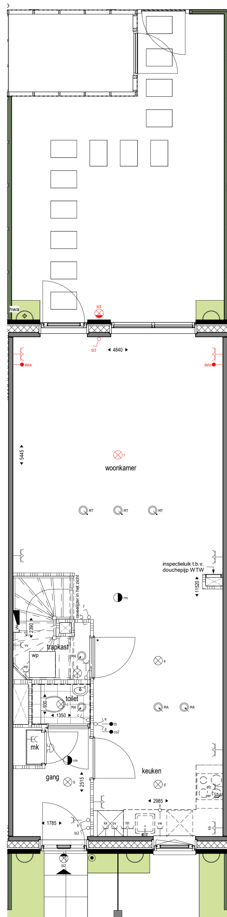
Begane grond 1 : 50
