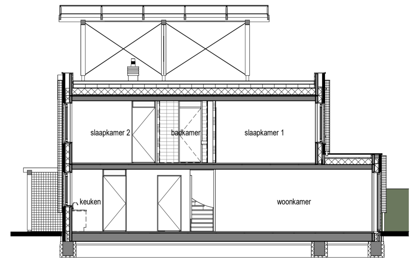
Doorsnede 1 : 100
