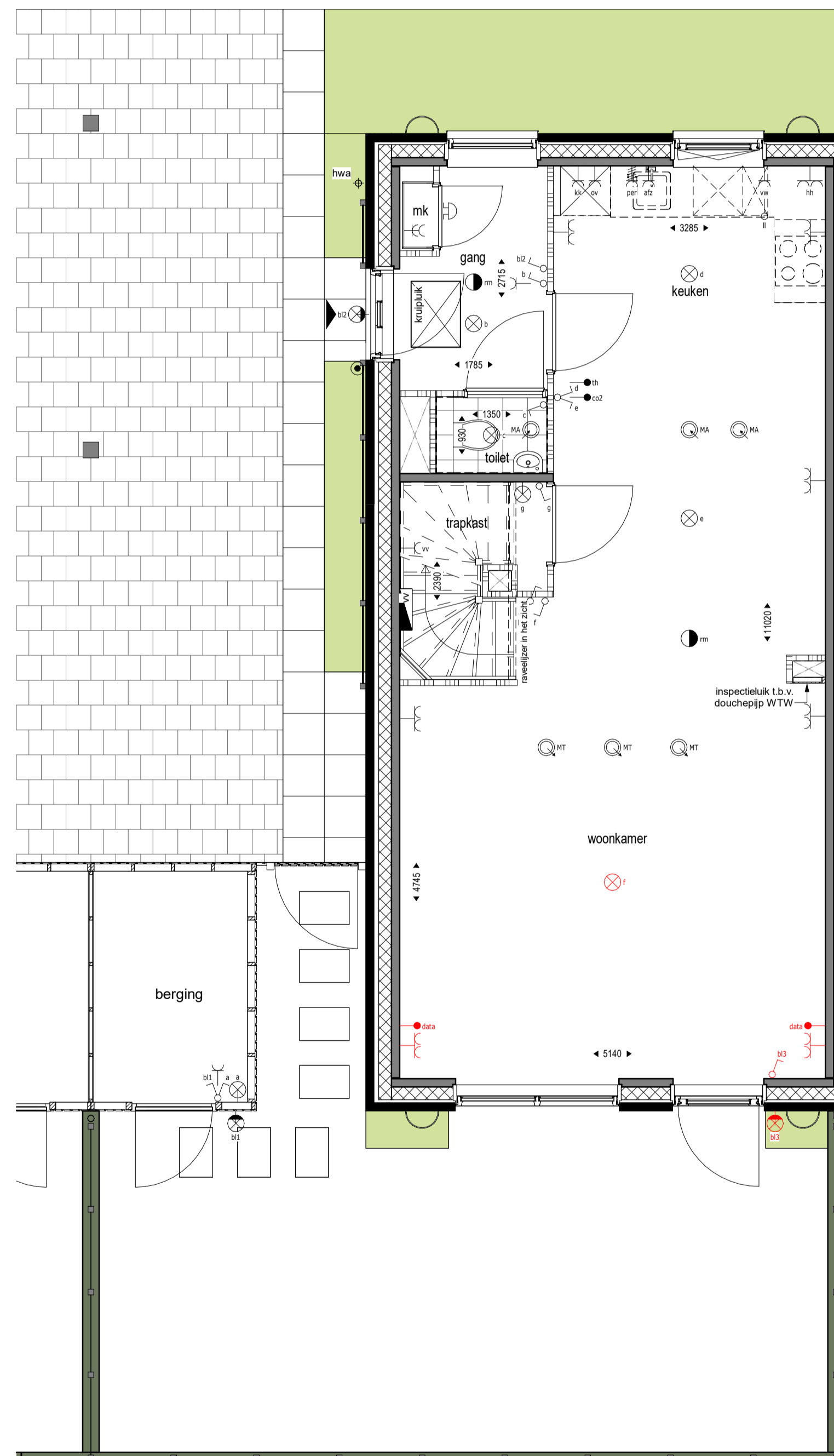
Begane grond 1 : 50
