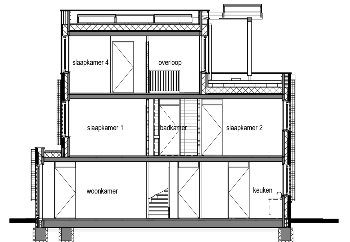
Doorsnede 1 : 100
