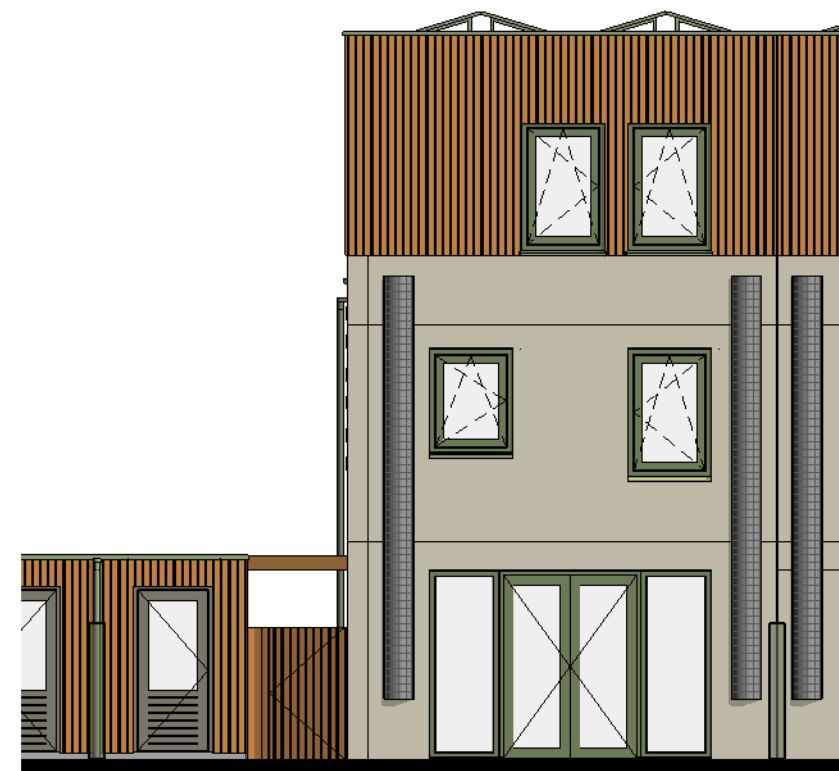
Achtergevel 1 : 100
