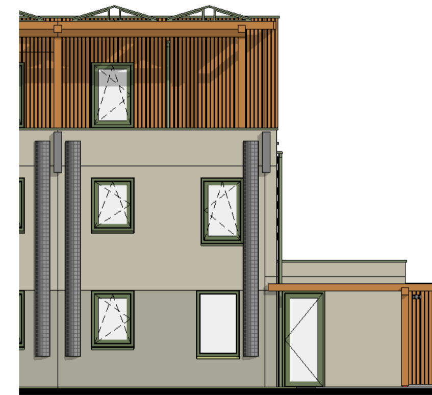
Voorgevel 1 : 100
