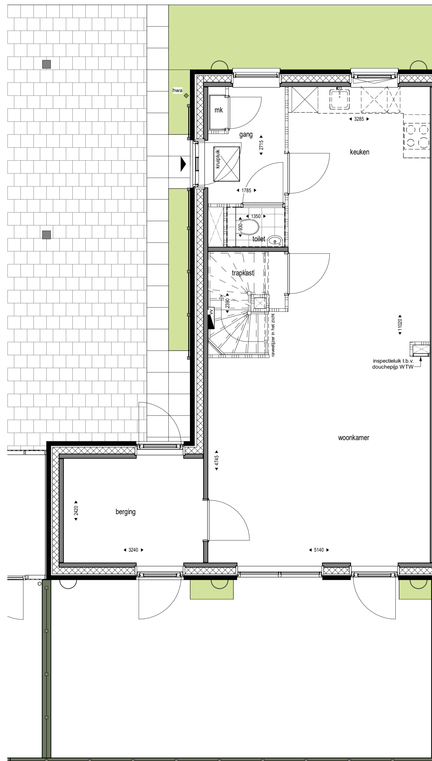
Begane grond 1 : 50
